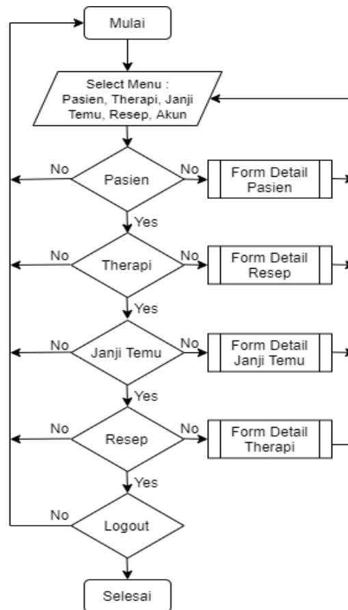
Gambar 4.2 Flowchart Aplikasi Rekam Medis Pasien
